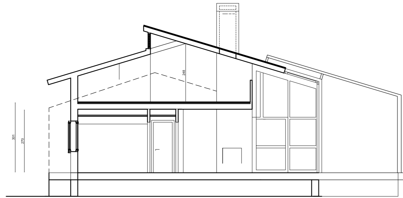
SEZIONE A-A
