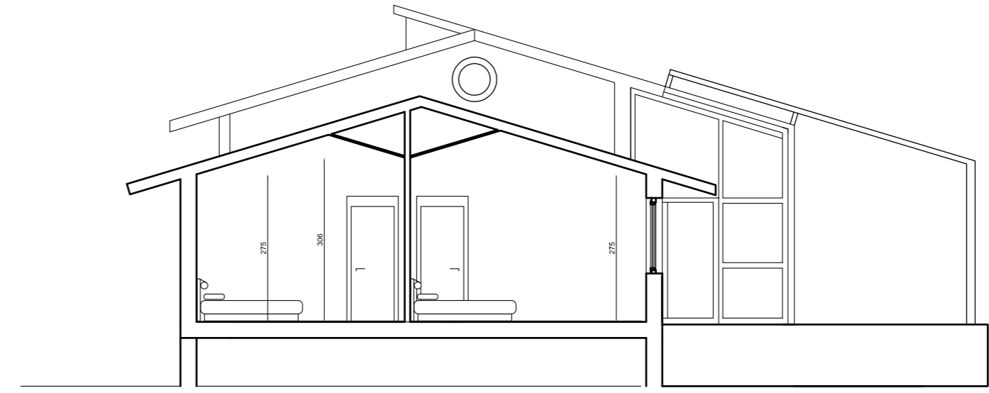
SEZIONE B-B
