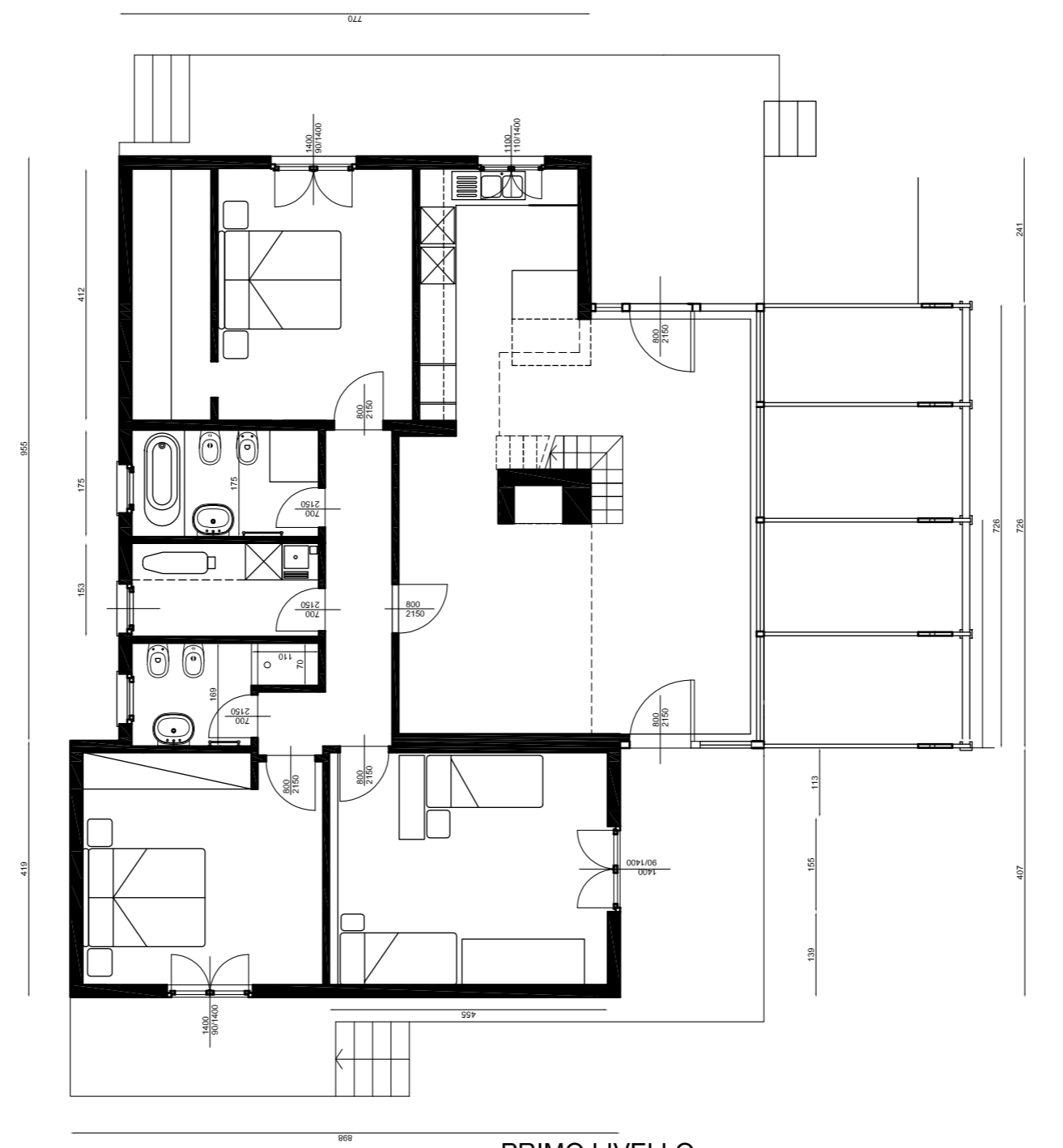
PRIMO LIVELLO
